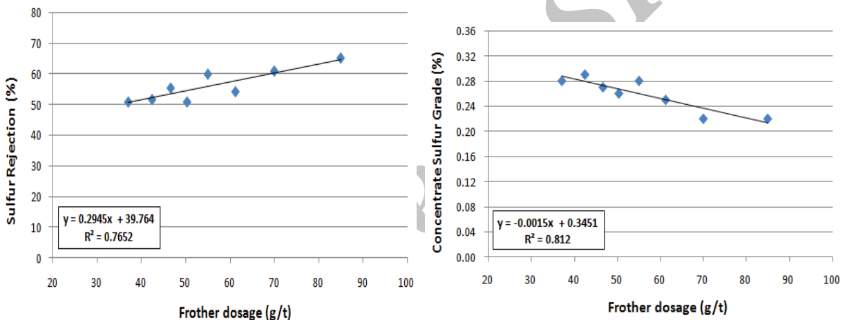
شکل ۶: تاثیر غلظت کفساز بر بازیابی و عیار گوگرد کنسانتره مدار فلوتاسیون
