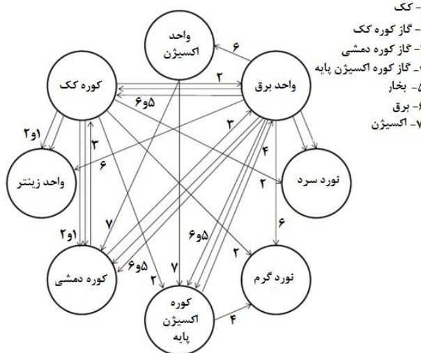
شکل ۲۰: جریان انرژی در واحدهای تولید فولاد متمرکز
