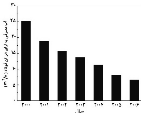
شکل ۱۶: آب مصرفی تازه به ازای هر تن فولاد [۱۷]
