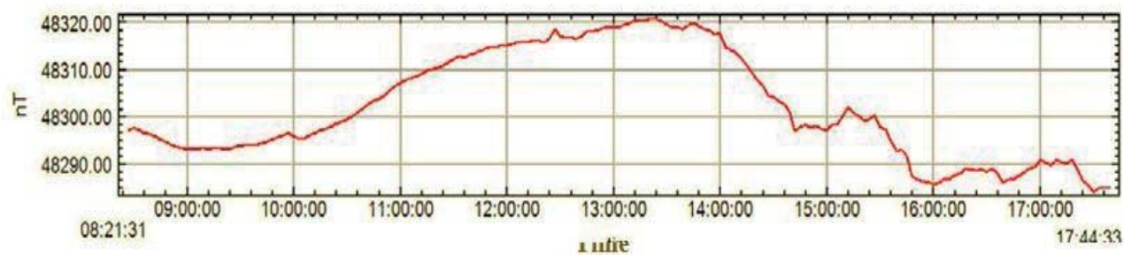
شکل ۲. تغییرات شدت میدان مغناطیسی در ایستگاه مینا در محدوده اکتشافی کلاته ناصر
