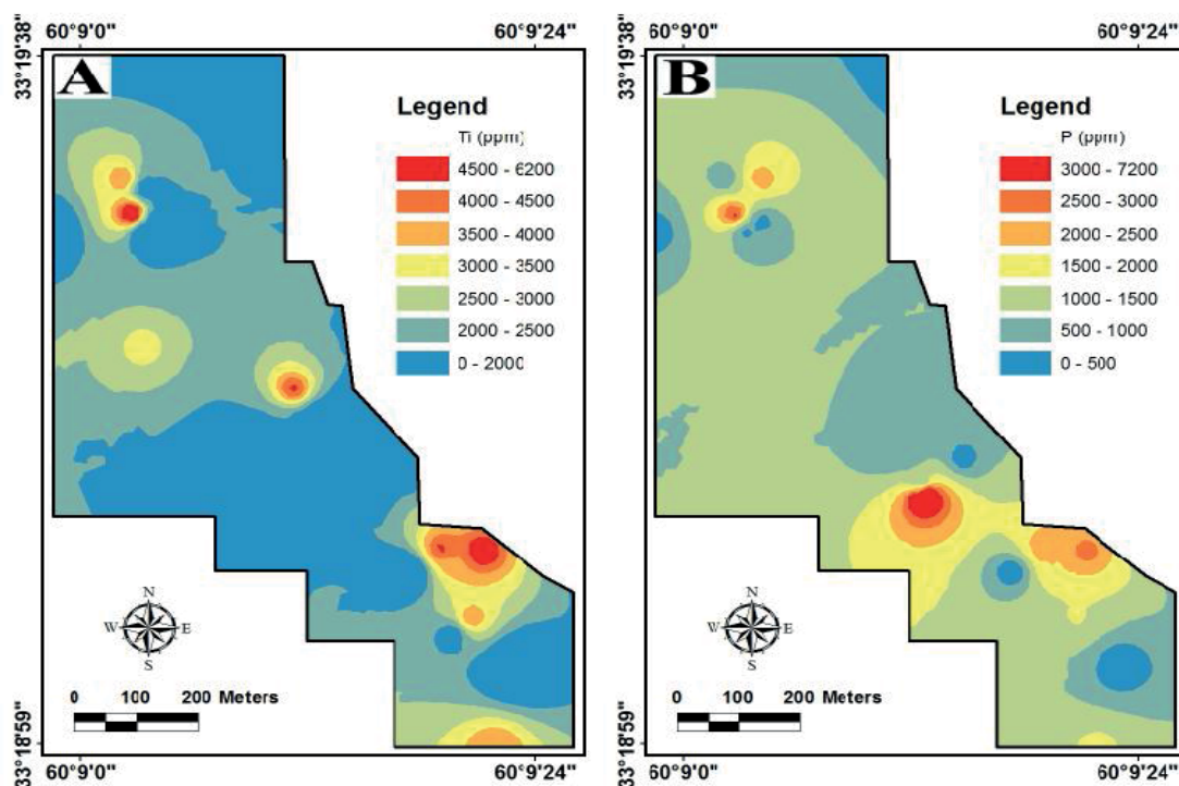
شکل ۸. نقشه توزیع ژئوشیمیایی A: عنصر تیتانیوم و B: عنصر فسفر در محدوده کلاته ناصر
