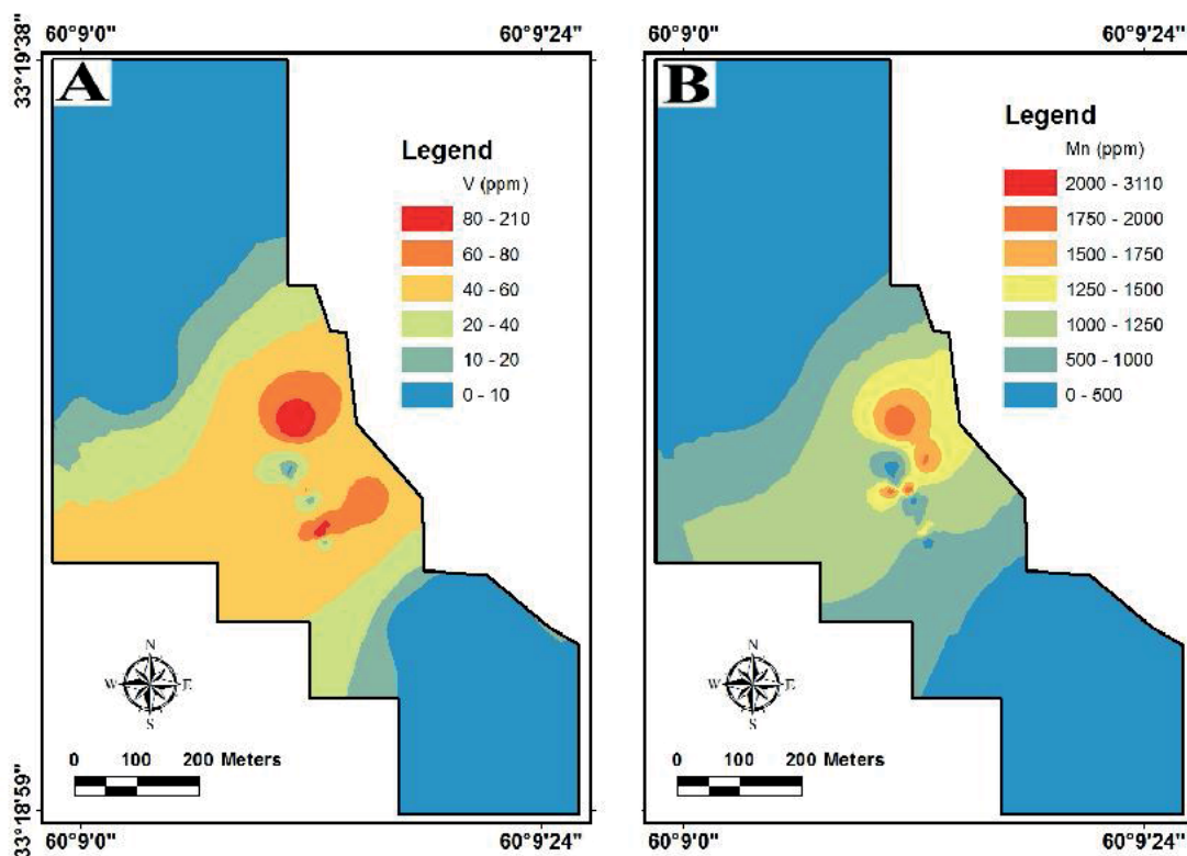
شکل ۹. نقشه توزیع ژئوشیمیایی A: عنصر وانادیوم و B: عنصر منگنز در محدوده کلاته ناصر
